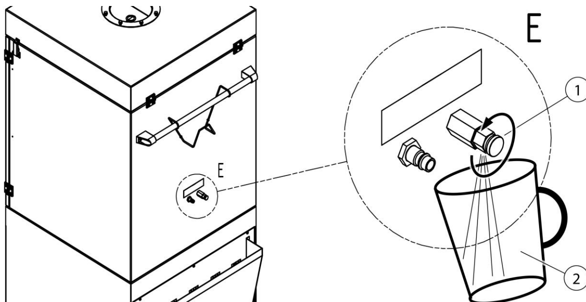
Afb. 8: Condensaat aftappen
