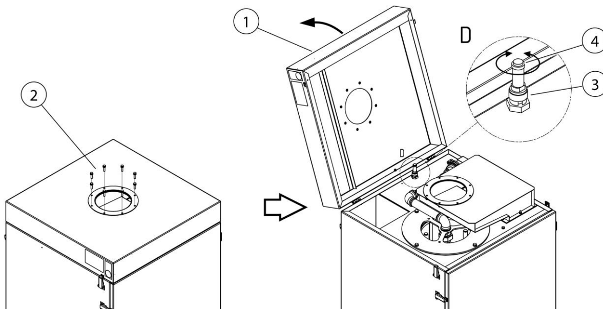
Afb. 12: Toegang tot het persluchtveiligheidsventiel
