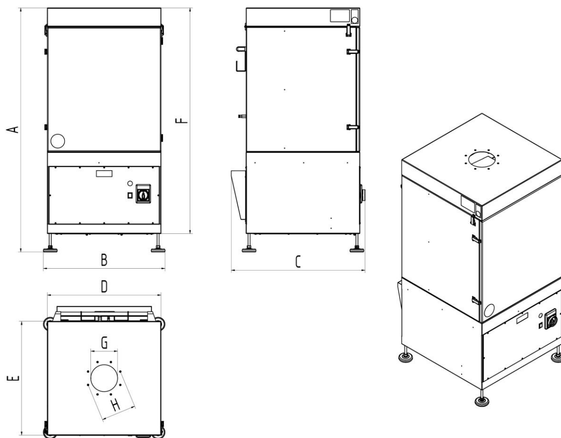
Afb. 13: Maatblad
