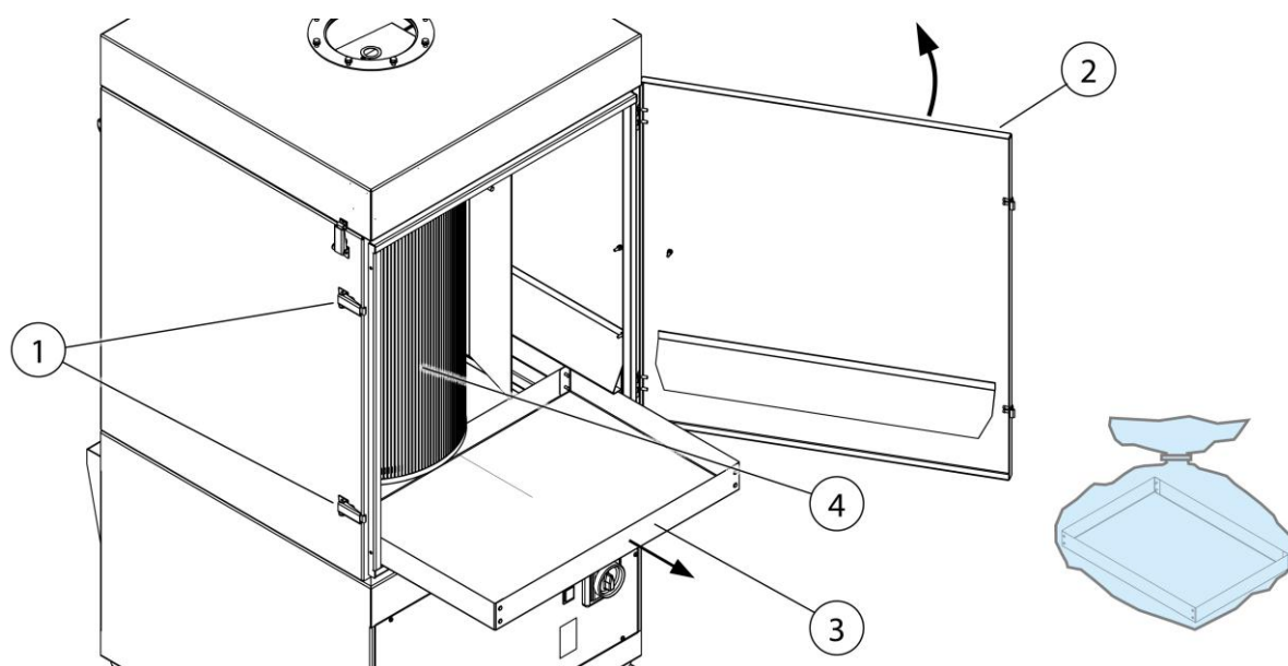
Afb. 7: Ledigen van het stofopvangreservoir
