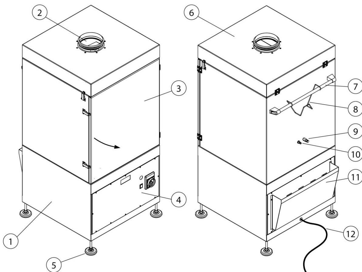
Afb. 1: Functiebeschrijving
